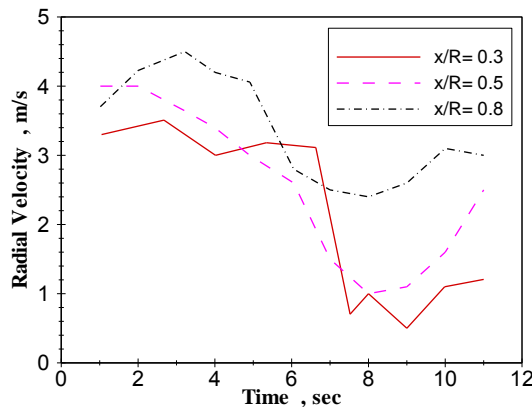
شکل ۱ - تغییرات سرعت شعاعی نسبت به زمان (B Nazanin ۱۲ pt, Bold) (فونت: B Nazanin, اندازه فونت ۱۲ و ضخیم) ۳۰ mm
